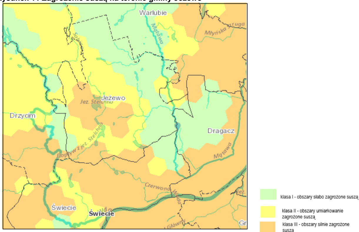
Rysunek 11 Zagrożenie suszą na terenie gminy Jeżewo
